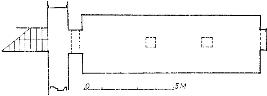
3. ábra: Szerdahely (Kaposzserdahely), a kolostor helyén álló pince alaprajza. Guzsik Tamás felmérése és rajza. (E könyv szerzője szerint ez a pince a török utáni újratelepülést követően készült a volt kolostor épületanyagából.)
